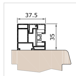
Vodicí lišta FS Z37VP, zaomitací varianta
