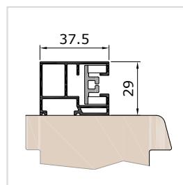
Standardní vodicí lišta FS Z37V
