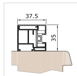
Standardní vodicí lišta FS Z37VS
