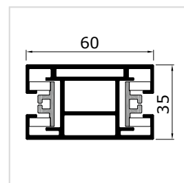
Odsazená vodicí lišta na sloupek FS ZT60VT
