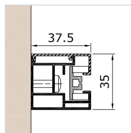
Vodicí lišta FS ZG37VS, montáž do ostění
