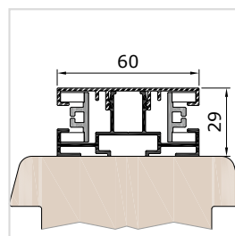
Vodicí lišta na sloupek FS ZT60V
