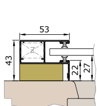
Termicky oddělená vodicí lišta K53VT
