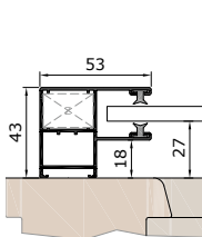
Vodicí lišta KA53V
