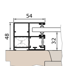
Vodicí lišta KR54V
