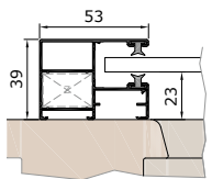
Vodicí lišta KF53V
