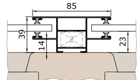
Sloupek s vodicí lištou KE85V
