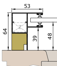
Termicky oddělená vodicí lišta KD53VT
