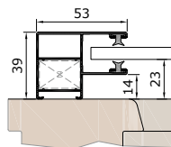
Vodicí lišta KE53V pro renovace
