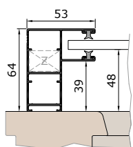
Vodicí lišta KD53V
