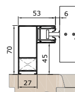
Vodicí lišta ED53V
