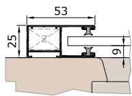
Vodicí lišta K53V
